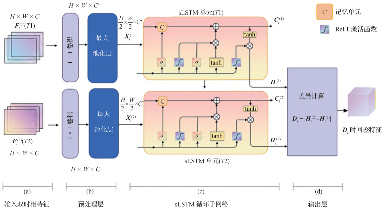
图2 时间存储器模块示意图
