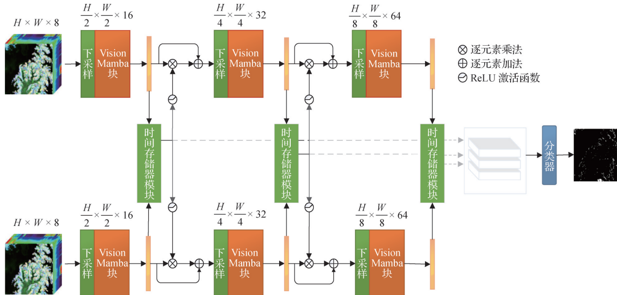
图1 时间差异引导网络整体框架图
